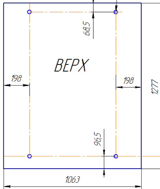
Рис.35А Места установки футорок на щитах декоративных (1200)
