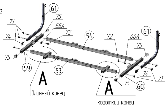
Рис.22.2 Положение штанги поз.53 при установке стола справа
