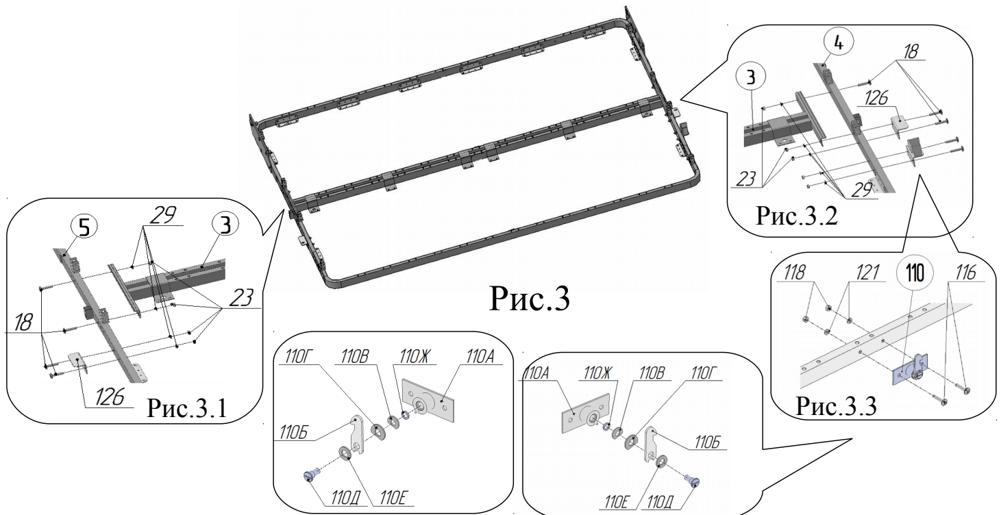
Рис 3.3.1 Фиксатор в сборе поз.110 для установки слева
